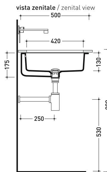
sezione longitudinale / section
