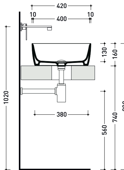
1020 sezione longitudinale / section
