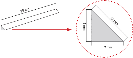
Sezione - Section
