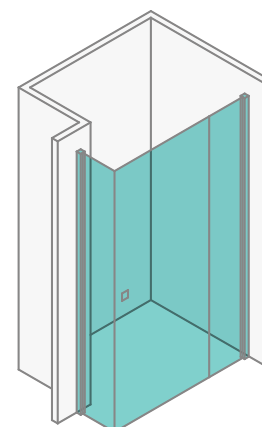
Монтаж профиля к торцу стены
